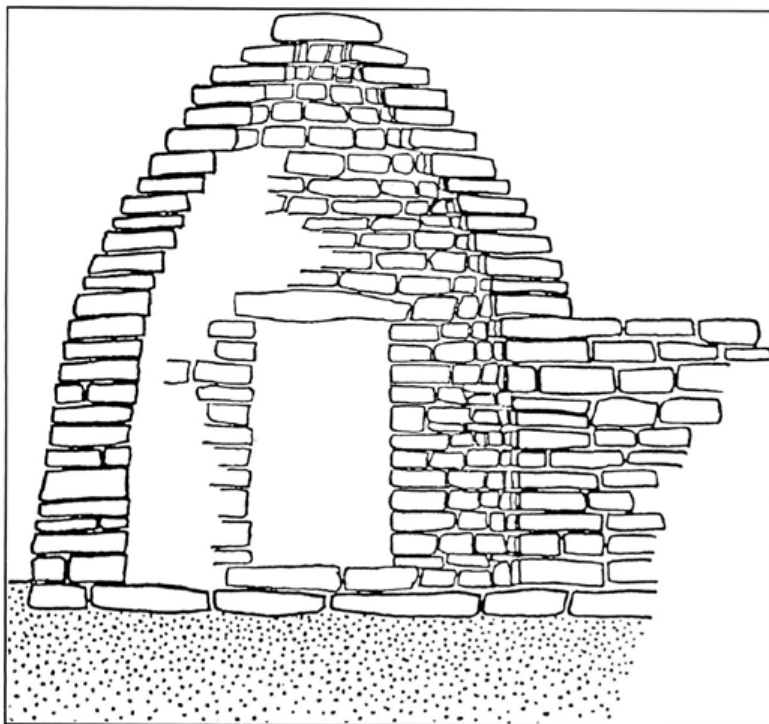
Coupe schématique d'une fausse voûte (Dessin : Daniel Marcelin)
